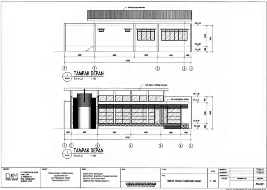
Gambar 59 Tampak Depan gedung kantor dan laboratorium UPTD Metrologi Legal Kabupaten/Kota Model B.
