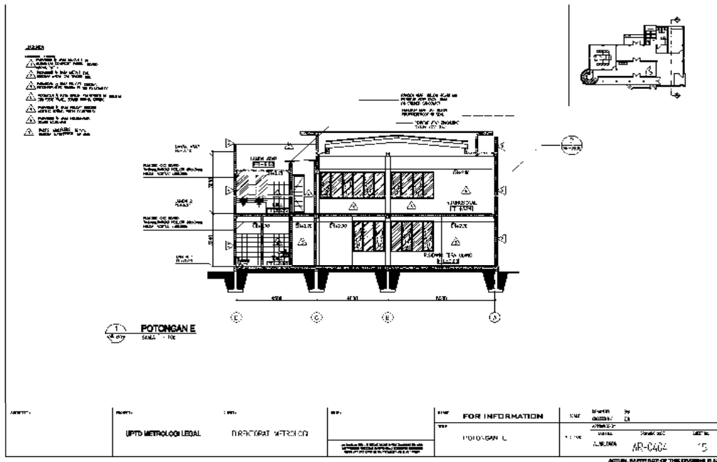
Gambar 35 Denah potongan E gedung kantor dan laboratorium UPTD Metrologi Legal Kabupaten/Kota Model A.
