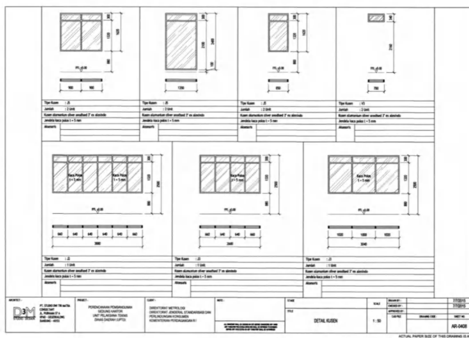
Gambar 68 Lanjutan Detail Kusen gedung kantor dan laboratorium UPTD Metrologi Legal Kabupaten/Kota Model B.
