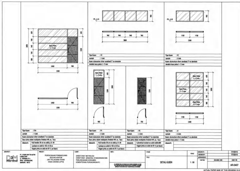
Gambar 67 Lanjutan Detail Kusen gedung kantor dan laboratorium UPTD Metrologi Legal Kabupaten/Kota Model B.
