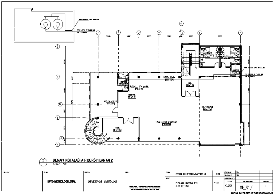
Gambar 47 Denah instalasi air bersih lantai 2 (dua) gedung kantor dan laboratorium UPTD Metrologi Legal Kabupaten/Kota Model A.
