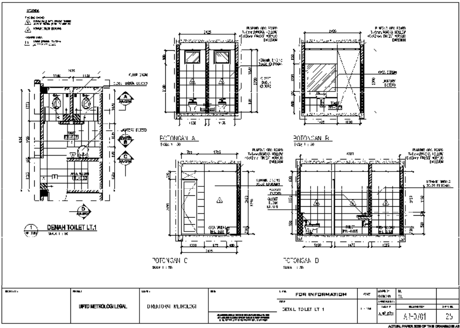
Gambar 45 Detail toilet lantai 1 (satu) gedung kantor dan laboratorium UPTD Metrologi Legal Kabupaten/Kota Model A.
