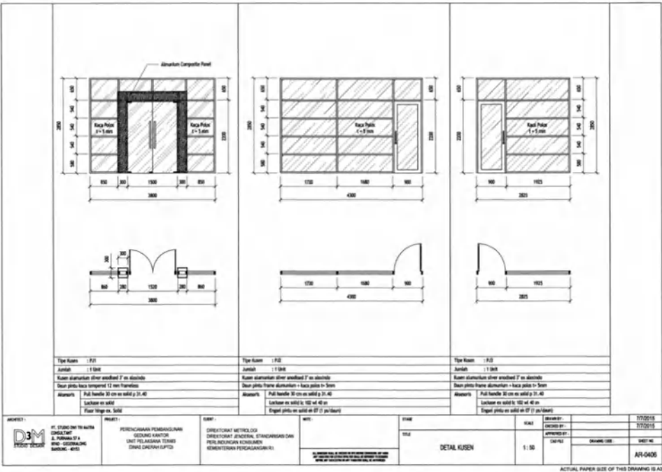
Gambar 65 Denah Schedule Kusen gedung kantor dan laboratorium UPTD Metrologi Legal Kabupaten/Kota Model
