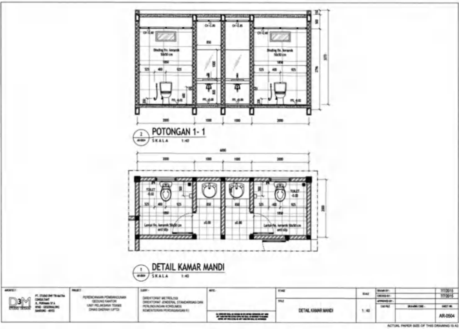
Gambar 70 Detail Kamar Mandi gedung kantor dan laboratorium UPTD Metrologi Legal Kabupaten/Kota Model B.
