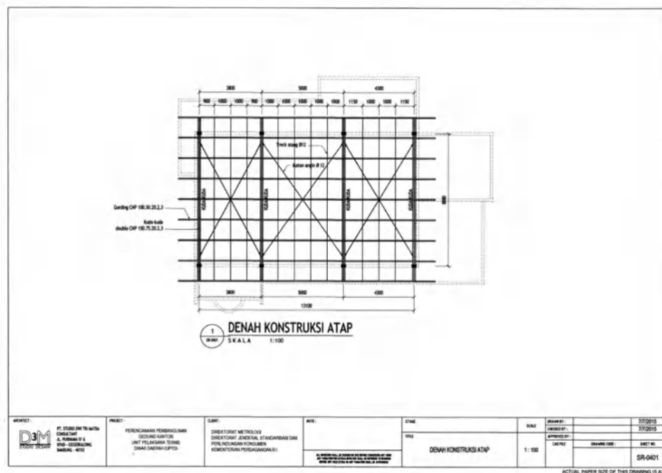
Gambar 78 Denah Konstruksi Atap gedung kantor dan laboratorium UPTD Metrologi Legal Kabupaten/Kota Model B.
