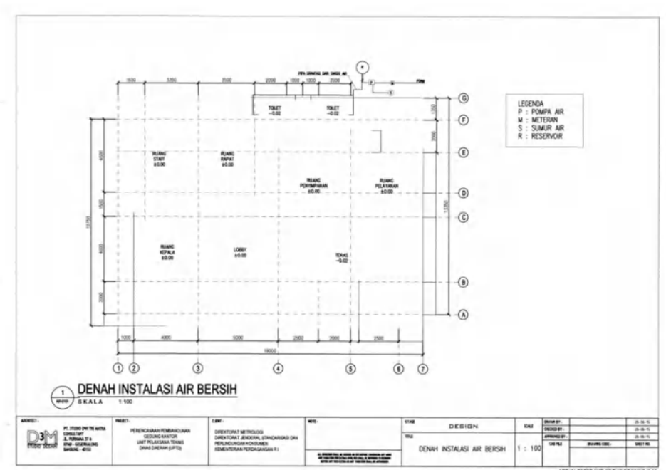
Gambar 71 Denah Instalasi Air Bersih gedung kantor dan laboratorium UPTD Metrologi Legal Kabupaten/Kota Model B.
