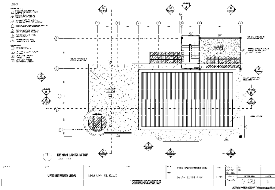
Gambar 25 Denah lantai atap gedung kantor dan laboratorium UPTD Metrologi Legal Kabupaten/Kota Model A.
