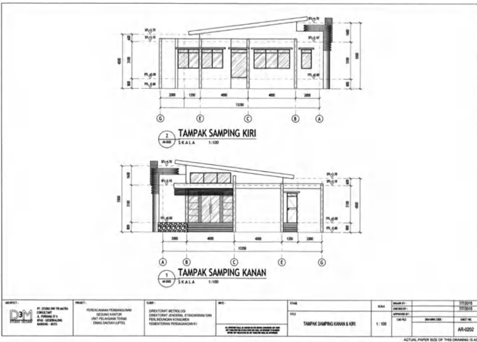
Gambar 60 Tampak samping kiri dan kanan gedung kantor dan laboratorium UPTD Metrologi Legal Kabupaten/Kota Model B.
