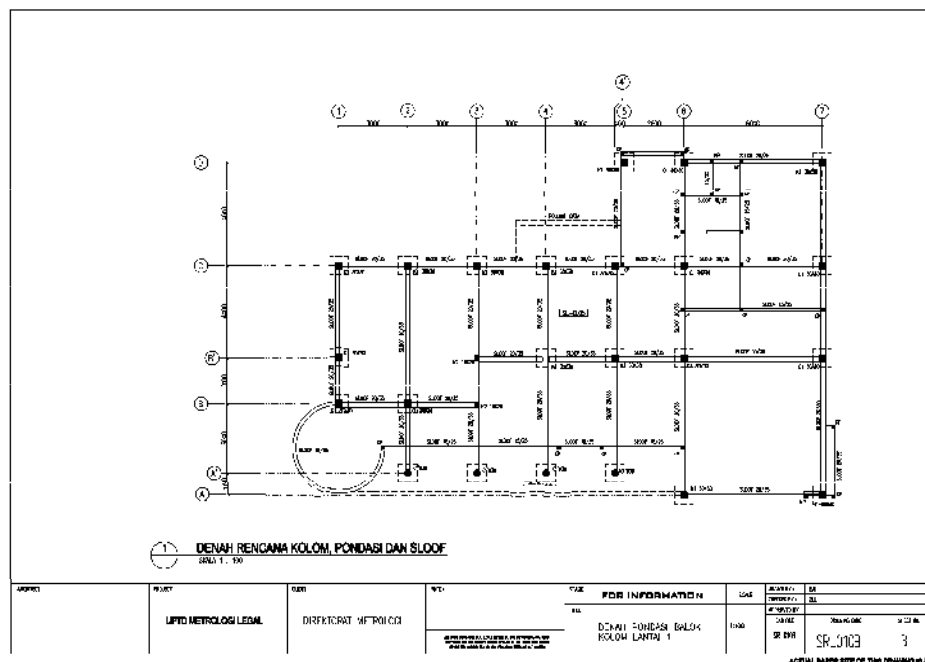
Gambar 55 Denah rencana kolom pondasi dan sloof gedung kantor dan laboratorium UPTD Metrologi Legal Kabupaten/Kota Model A.
