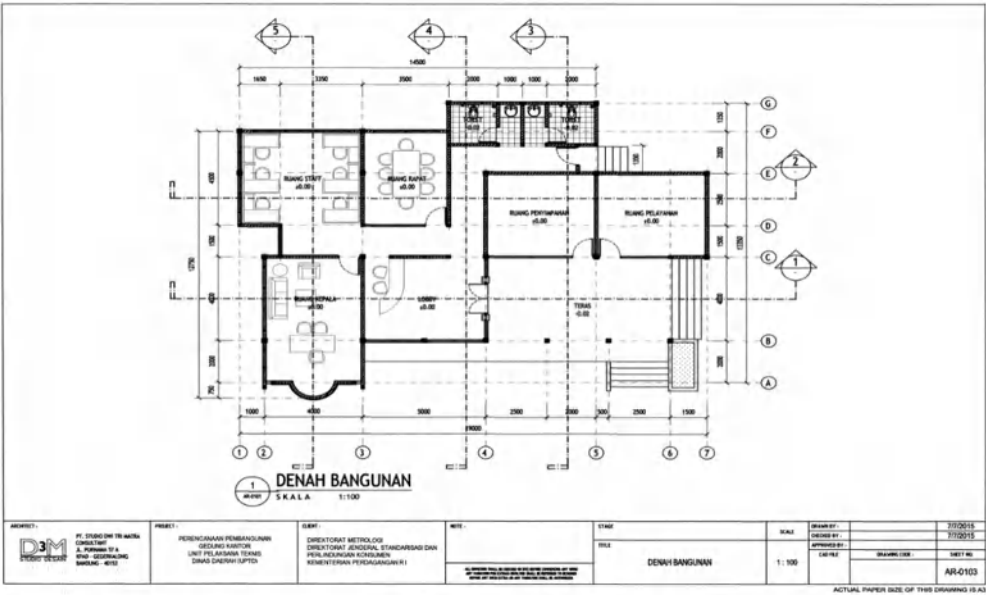
Gambar 57 Denah Bangunan gedung kantor dan laboratorium UPTD Metrologi Legal Kabupaten/Kota Model B.
