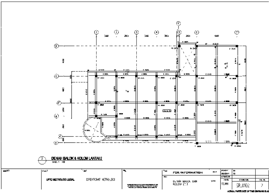
Gambar 54 Denah balok & kolom lantai 2 (dua) gedung kantor dan laboratorium UPTD Metrologi Legal Kabupaten/Kota Model A
