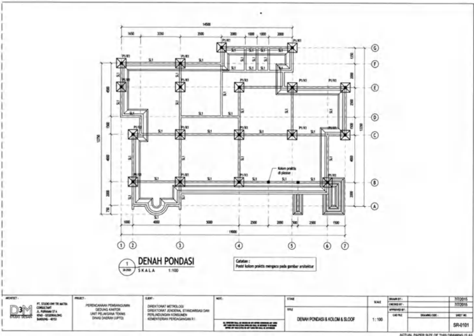
Gambar 74 Denah Pondasi gedung kantor dan laboratorium UPTD Metrologi Legal Kabupaten/Kota Model B.
