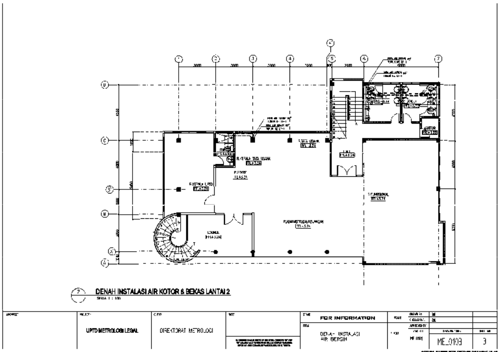
Gambar 48 Denah instalasi air kotor & bekas lantai 2 (dua) gedung kantor dan laboratorium UPTD Metrologi Legal Kabupaten/Kota Model A.
