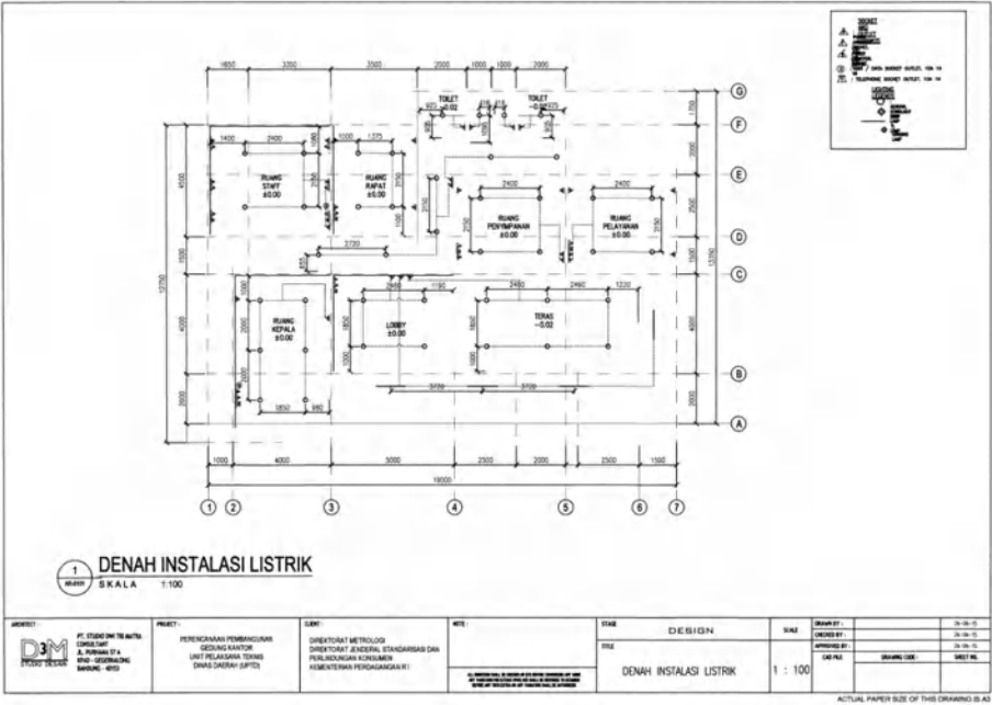
Gambar 73 Denah Instalasi Listrik gedung kantor dan laboratorium UPTD Metrologi Legal Kabupaten/Kota Model B.
