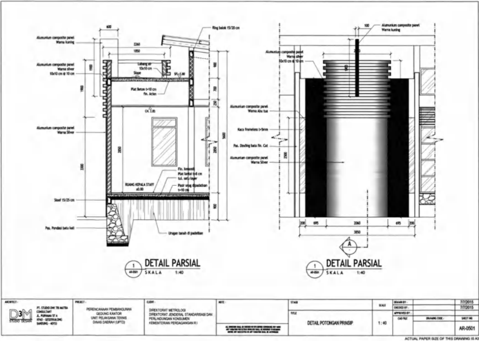
Gambar 69 Detail Potongan Prinsip gedung kantor dan laboratorium UPTD Metrologi Legal Kabupaten/Kota Model B.
