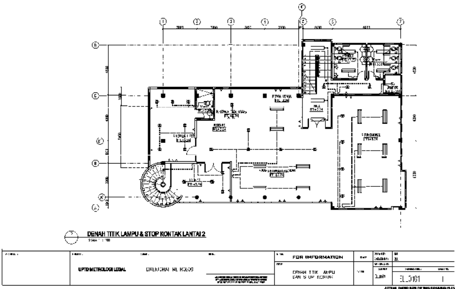
Gambar 49 Denah titik & stop kontak lantai 2 (dua) gedung kantor dan laboratorium UPTD Metrologi Legal Kabupaten/Kota Model A.
