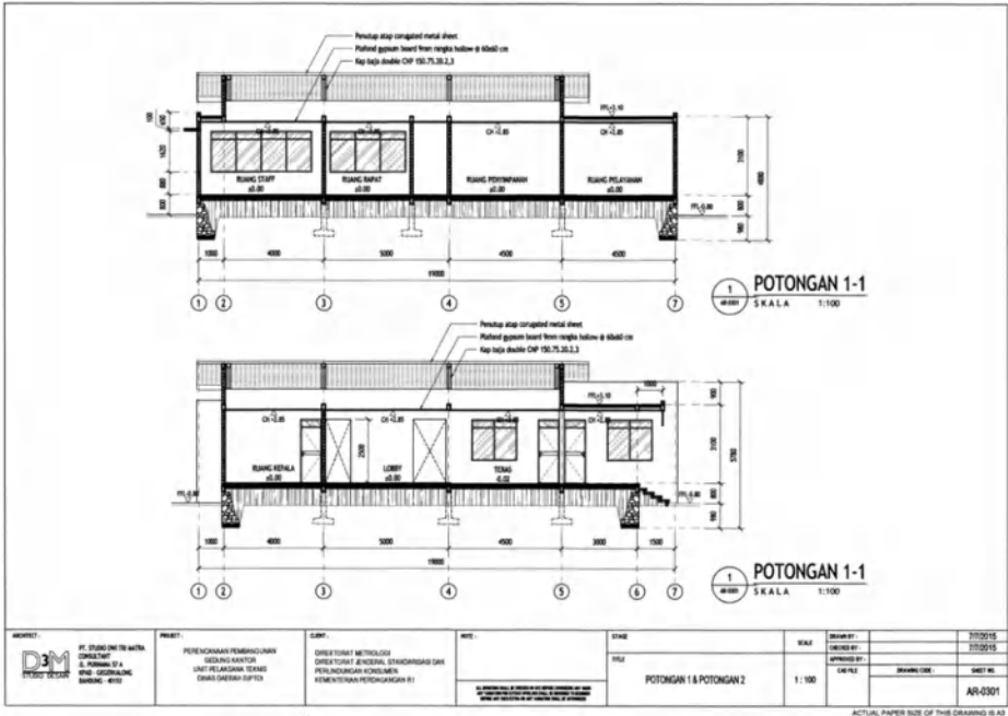
Gambar 61 Potongan 1-1 gedung kantor dan laboratorium UPTD Metrologi Legal Kabupaten/Kota Model B.
