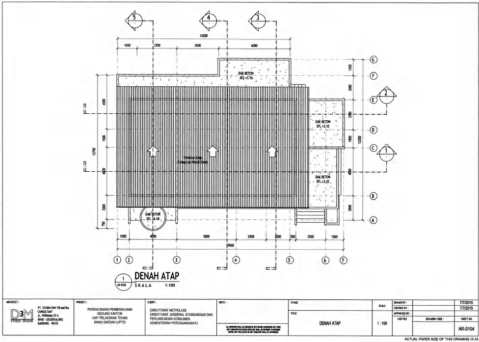
Gambar 58 Denah Atap gedung kantor dan laboratorium UPTD Metrologi Legal Kabupaten/Kota Model B.
