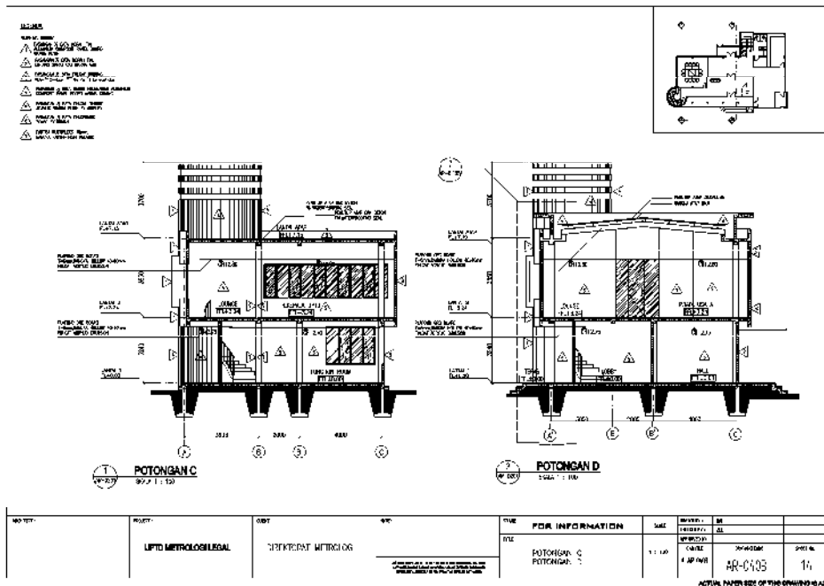
Gambar 34 Denah potongan C dan D gedung kantor dan laboratorium UPTD Metrologi Legal Kabupaten/Kota Model A.
