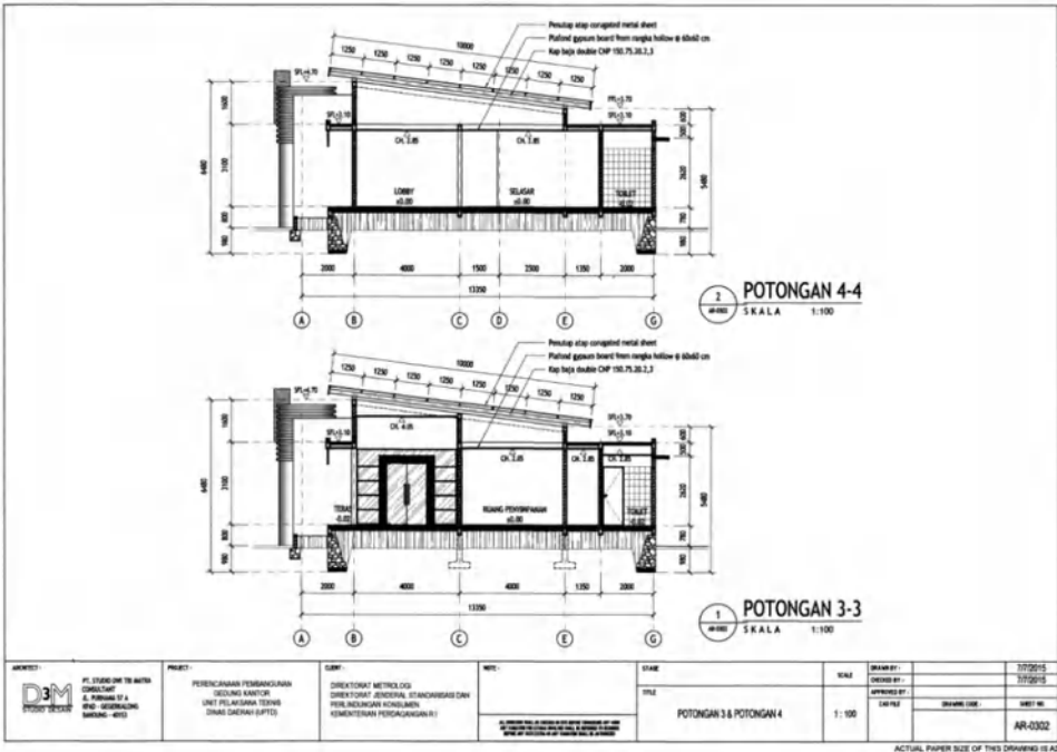
Gambar 62 Potongan 3-3 gedung kantor dan laboratorium UPTD Metrologi Legal Kabupaten/Kota Model B.
