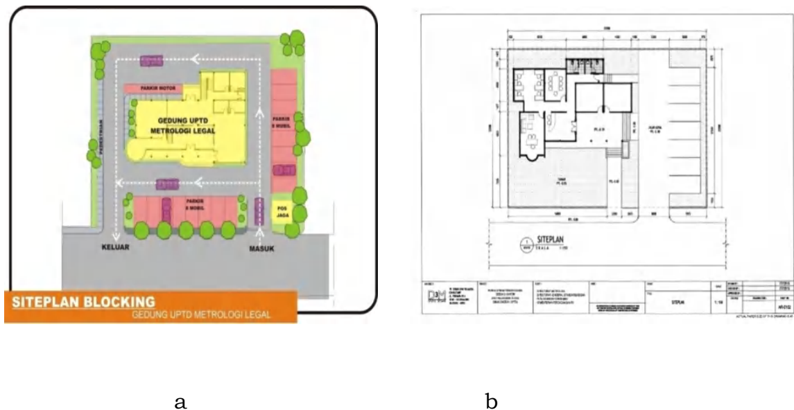
Gambar 18 Contoh Siteplan Blocking Gedung Kantor dan Laboratorium UPTD Metrologi Legal Kabupaten/Kota: a) Model A; b) Model B
