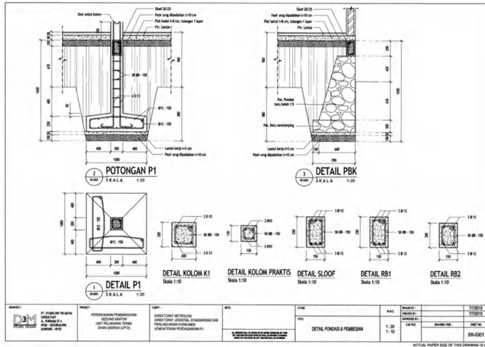
Gambar 77 Detail Pondasi & Pembesian gedung kantor dan laboratorium UPTD Metrologi Legal Kabupaten/Kota Model B.
