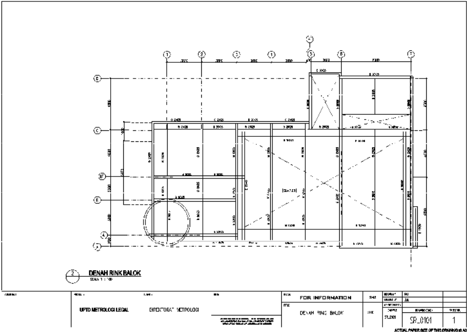
Gambar 53 Denah ring balok gedung kantor dan laboratorium UPTD Metrologi Legal Kabupaten/Kota Model A.
