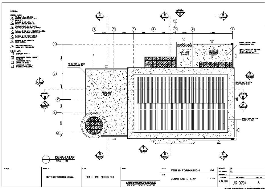
Gambar 26 Denah atap gedung kantor dan laboratorium UPTD Metrologi Legal Kabupaten/Kota Model A.
