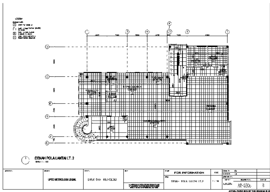
Gambar 28 Denah pola lantai 2 (dua) gedung kantor dan laboratorium UPTD Metrologi Legal Kabupaten/Kota Model A.
