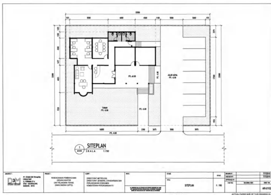
Gambar 56 Denah Siteplan gedung kantor dan laboratorium UPTD Metrologi Legal Kabupaten/Kota Model B.
