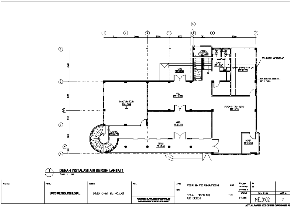
Gambar 50 Denah instalasi air bersih lantai 1 (satu) gedung kantor dan laboratorium UPTD Metrologi Legal Kabupaten/Kota Model A.
