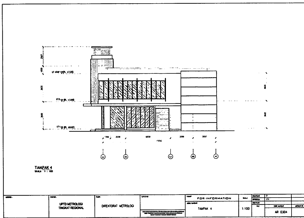
Gambar 44. Detail Tampak Samping 2 Gedung Kantor dan Laboratorium UPTD Metrologi Legal Provinsi.
