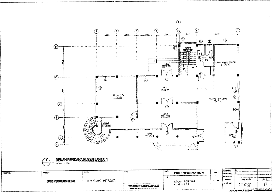
Gambar 17. Denah Rencana Kusen Lantai 1 Gedung Kantor dan Laboratorium UPTD Metrologi Legal Kabupaten/Kota.
