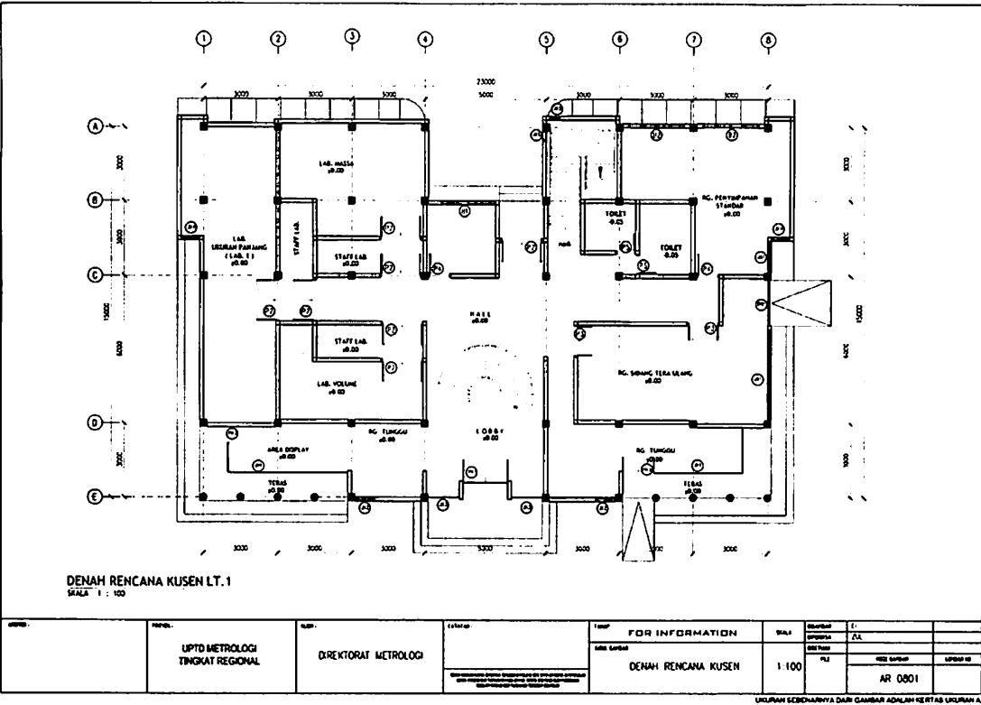
Gambar 55. Denah Rencana Kusen Gedung Kantor dan Laboratorium UPTD Metrologi Legal Provinsi.
