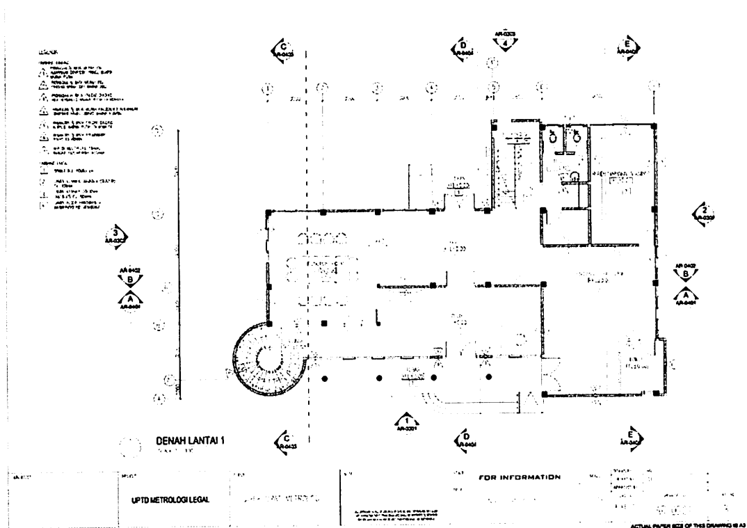
Gambar 3. Denah Lantai 1 Gedung Kantor dan Laboratorium UPTD Metrologi Legal Kabupaten/Kota.
