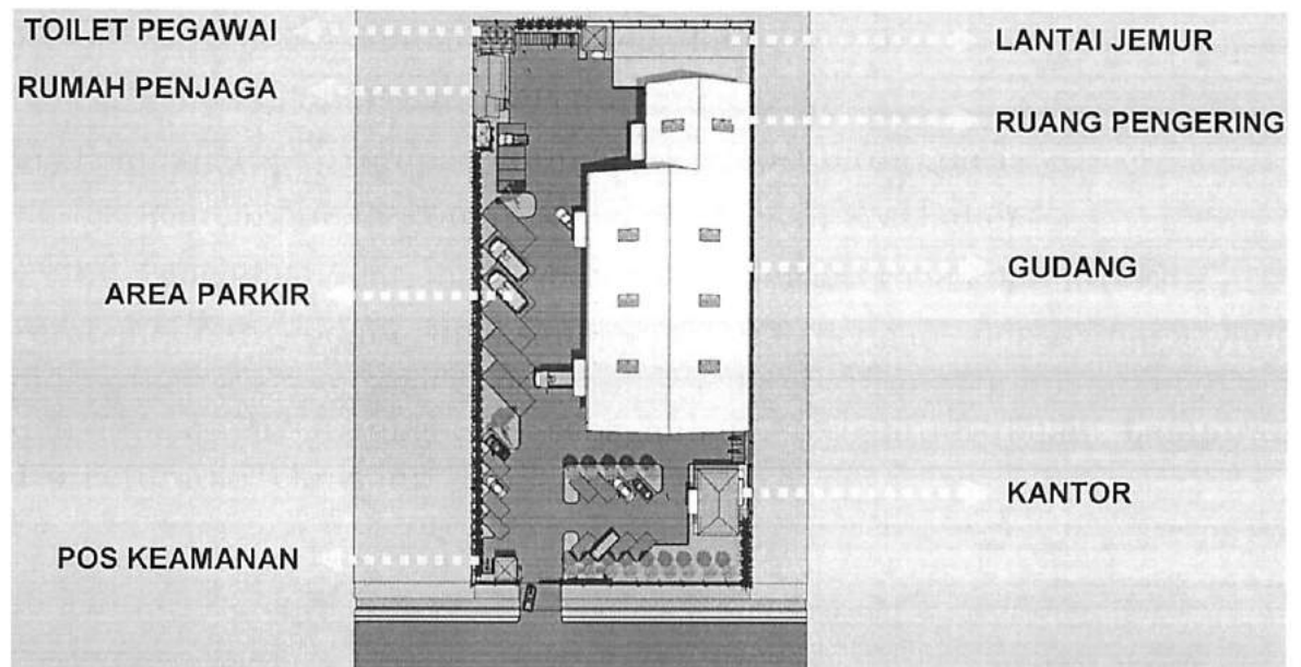
Gambar 9. Site Plan Gudang SRG Tampak Atas
