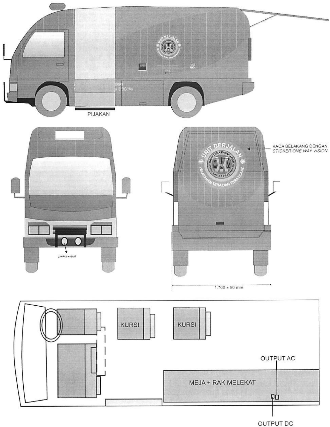
Gambar 18. Contoh Desain Unit Berjalan Pelayanan Tera dan Tera Ulang
