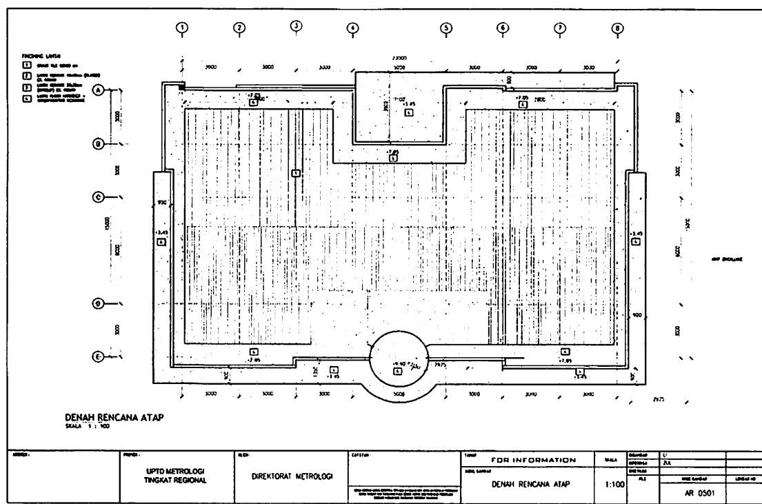
Gambar 50. Denah Rencana Atap Gedung Kantor dan Laboratorium UPTD Metrologi Legal Provinsi.
