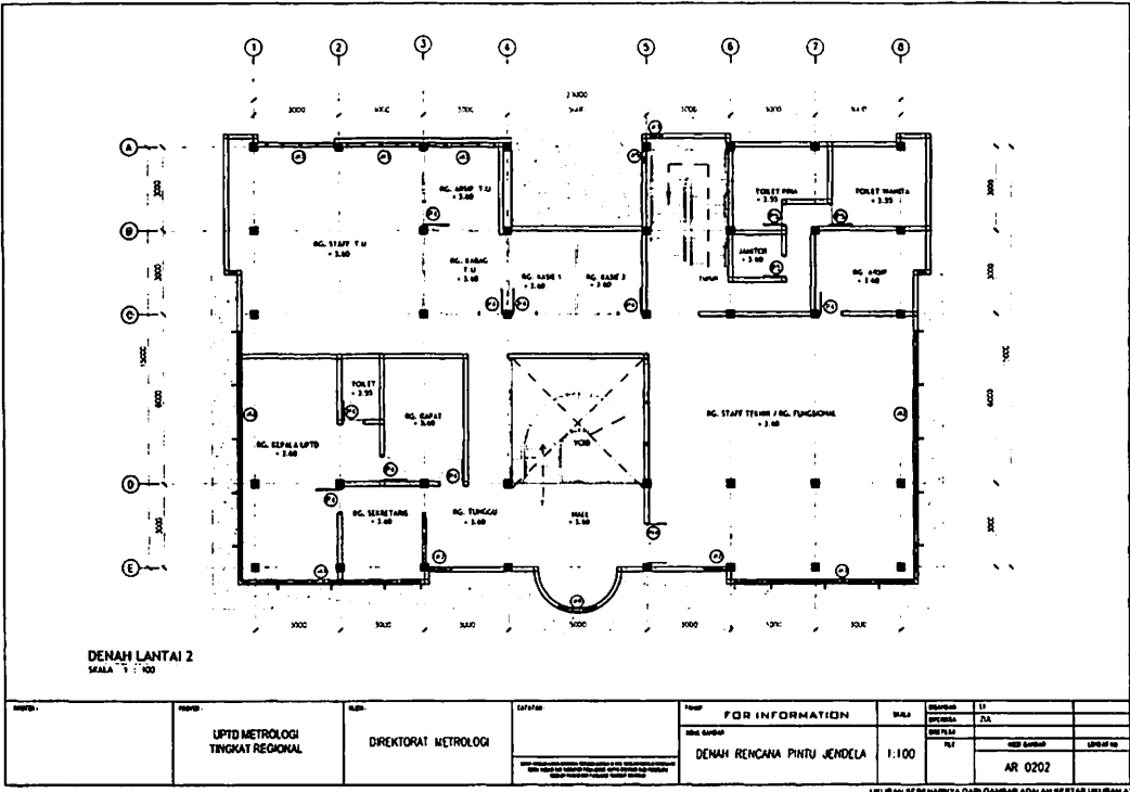
Gambar 56. Denah Rencana Pintu Jendela Gedung Kantor dan Laboratorium UPTD Metrologi Legal Provinsi.
