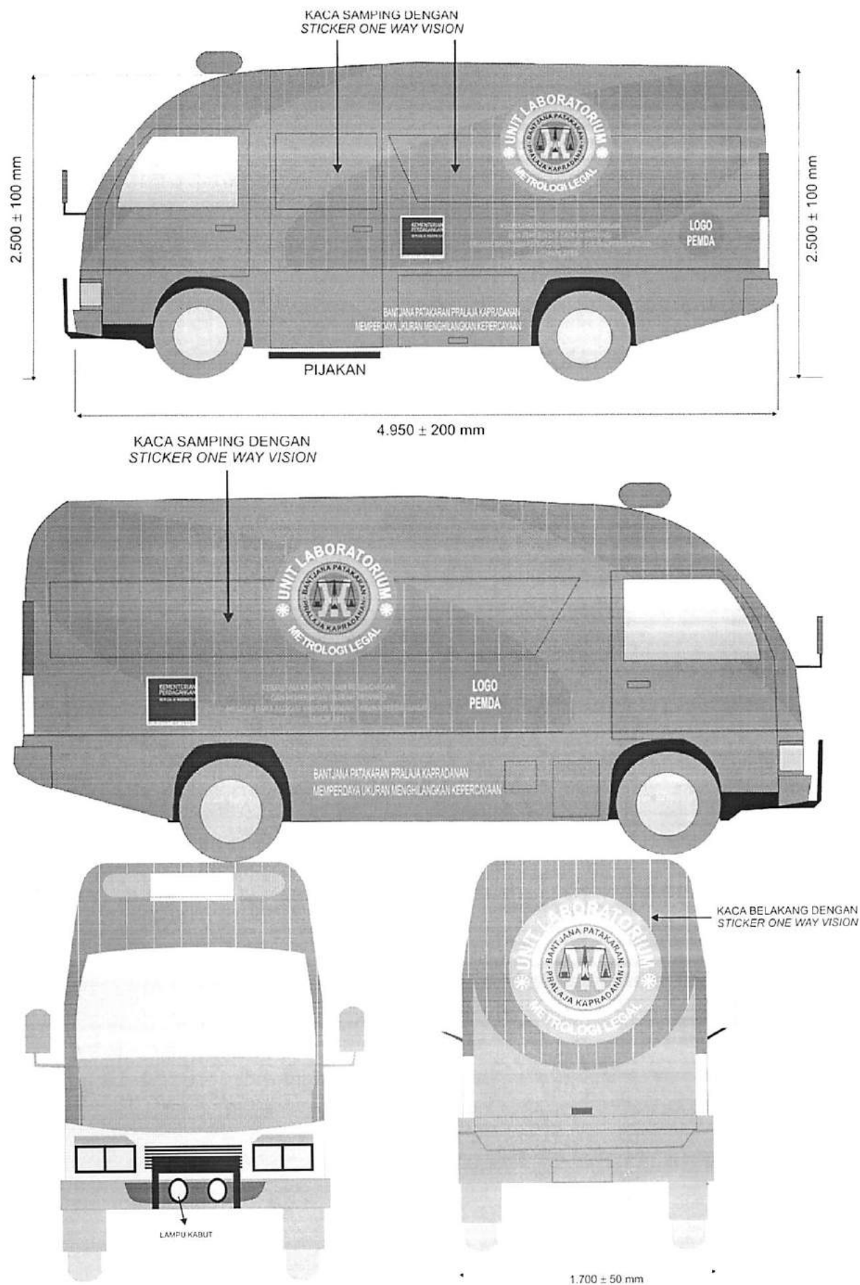
Gambar 28. Contoh Desain Unit Laboratorium Metrologi Legal Berjalan
