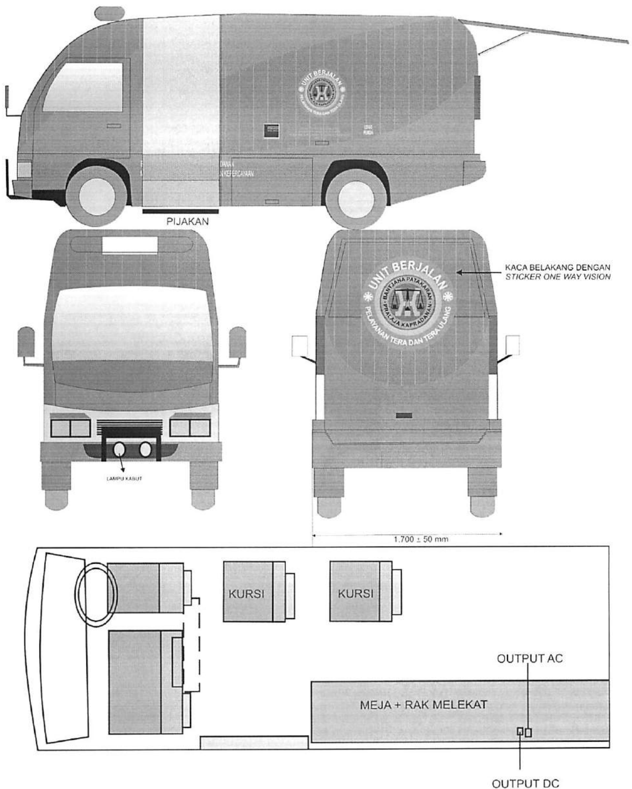
Gambar 30. Contoh Desain Unit Berjalan Pelayanan Tera dan Tera Ulang
