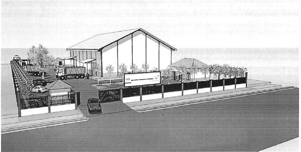
Gambar 10. Site Plan Gudang SRG Tampak Depan
