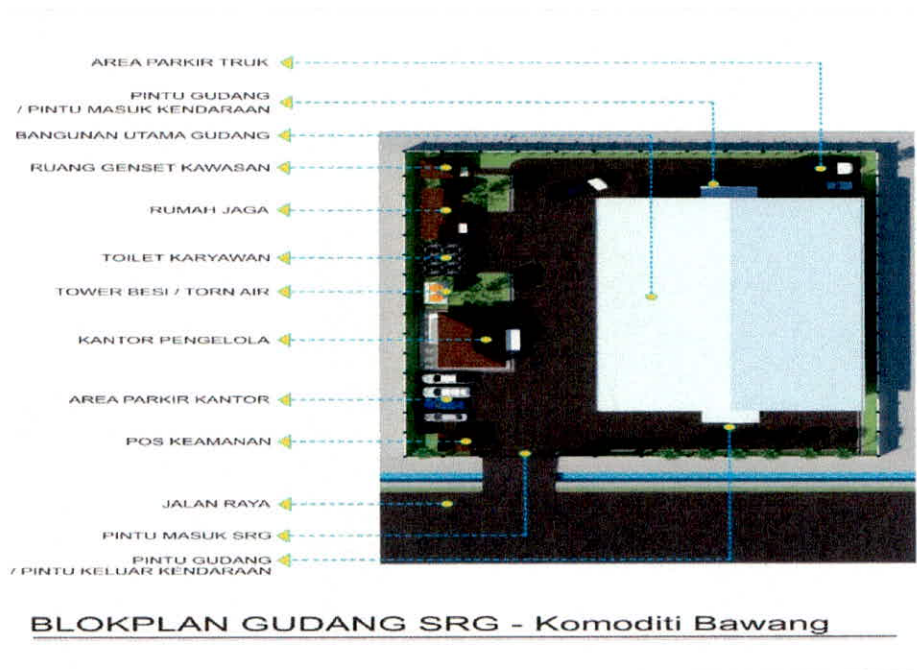
Gambar 5. Gudang SRG untuk Komoditi Bawang Merah Tampak Atas
