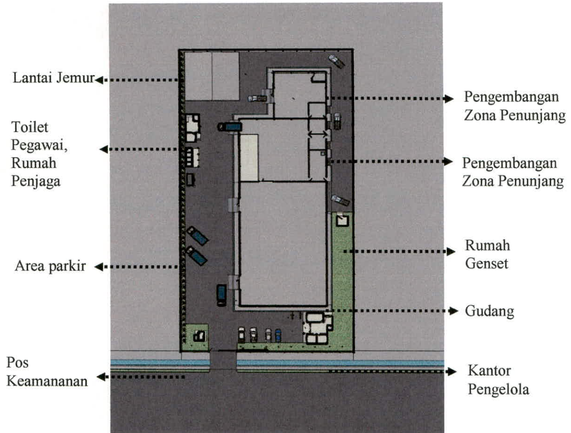
Gambar 1. Site Plan Gudang SRG Tampak Atas
